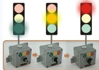
Selector de 3 posiciones Verde/Amarillo/Rojo
